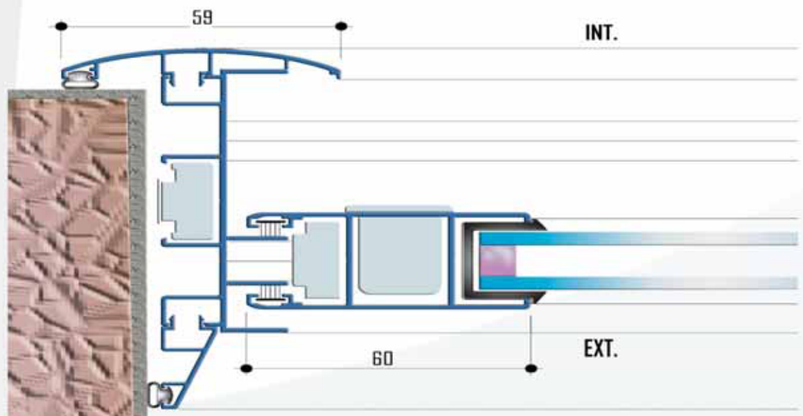
Coupe horizontale sur montant latéral
