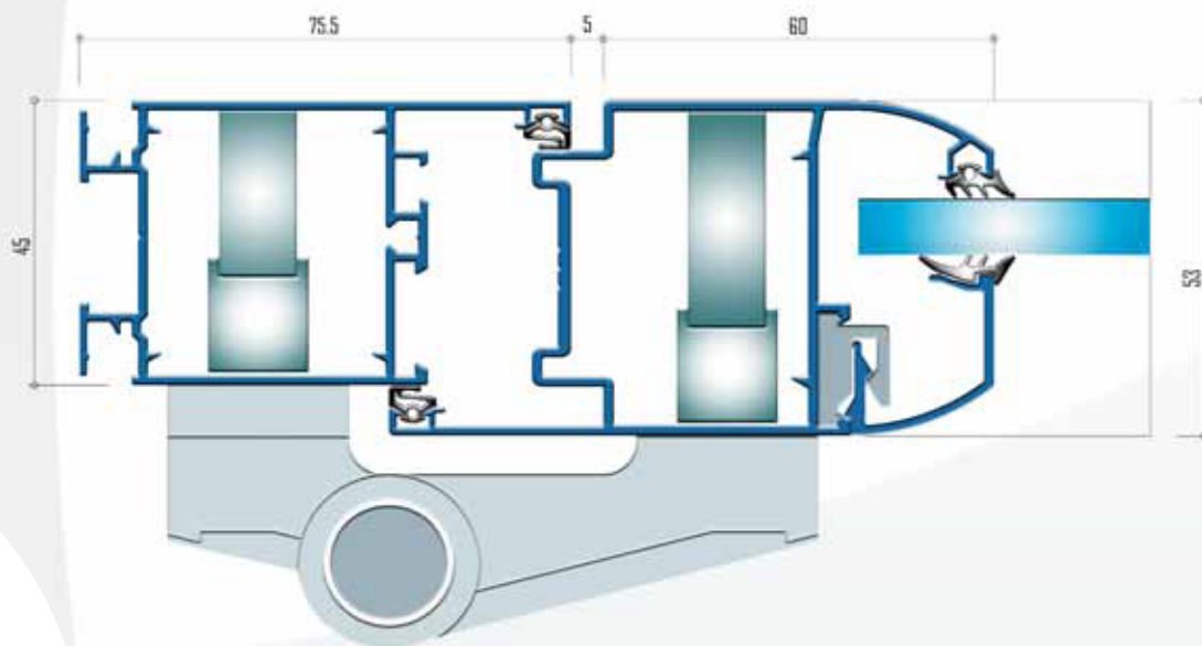
Coupe horizontale sur montant latéral
