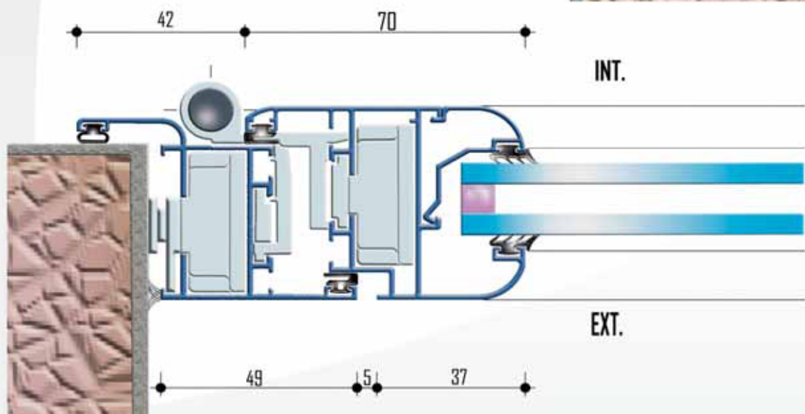
Coupe horizontale sur montant latéral
