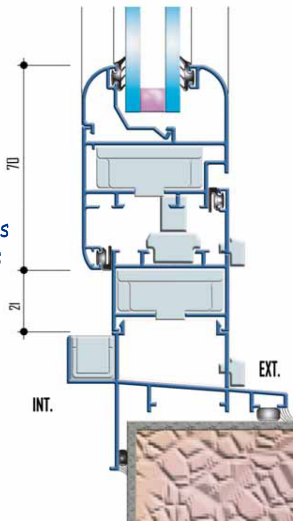
Coupe verticale sur traverse inférieure
