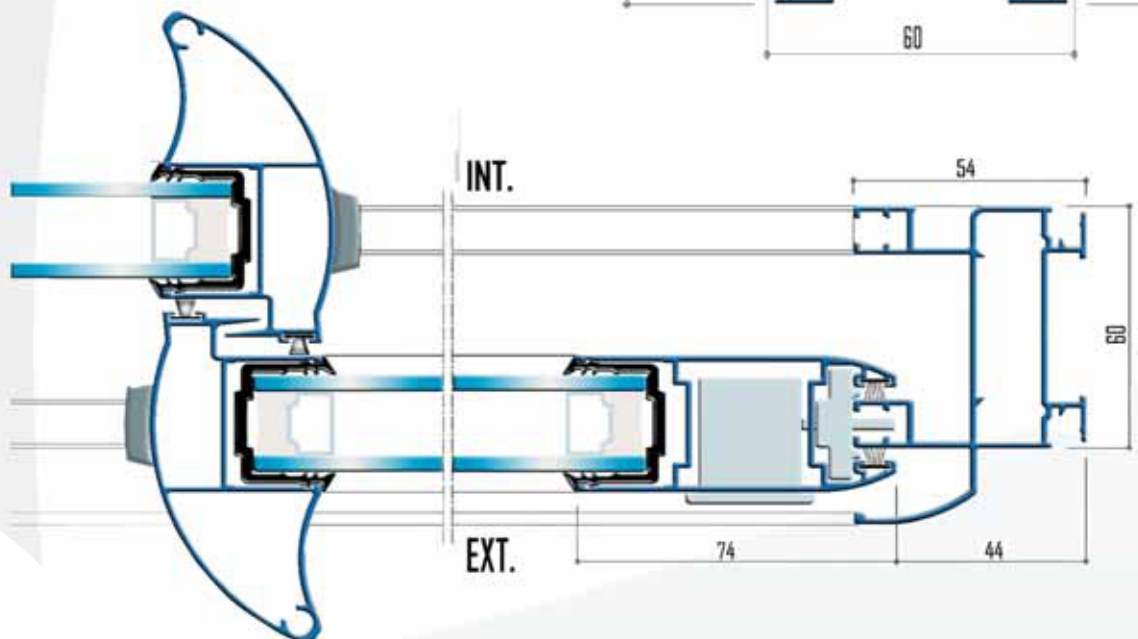
Coupe horizontale sur montant central et latéral
