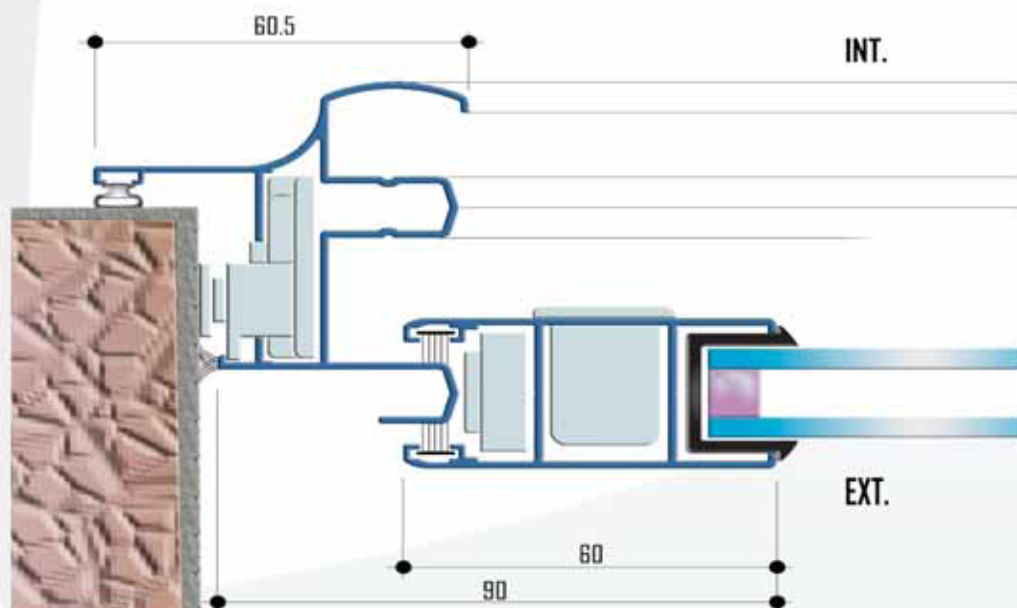
Coupe horizontale sur montant latéral
